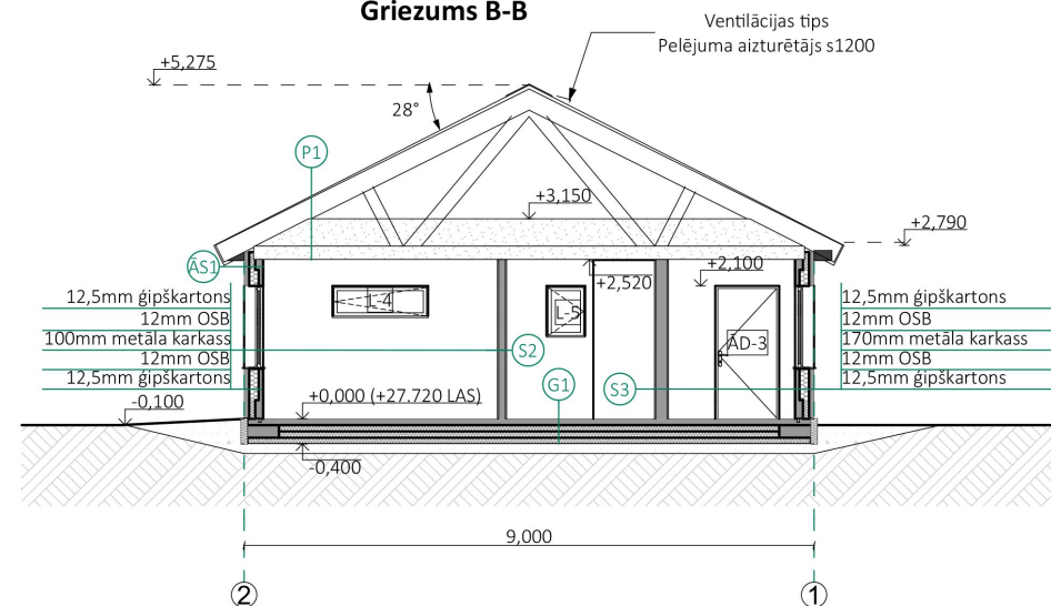
Griezums B-B
