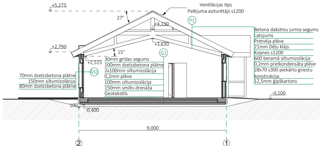
Griezums A-A
